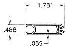
11 PERIMETER SPACER
